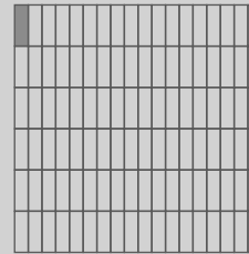
ITEM 2 Tessera size 1,5 x 4,7 cm · 5/8" x 1 7/8" Sheet size 29,6 x 29,6 cm · 11 5/8" x 11 5/8"
